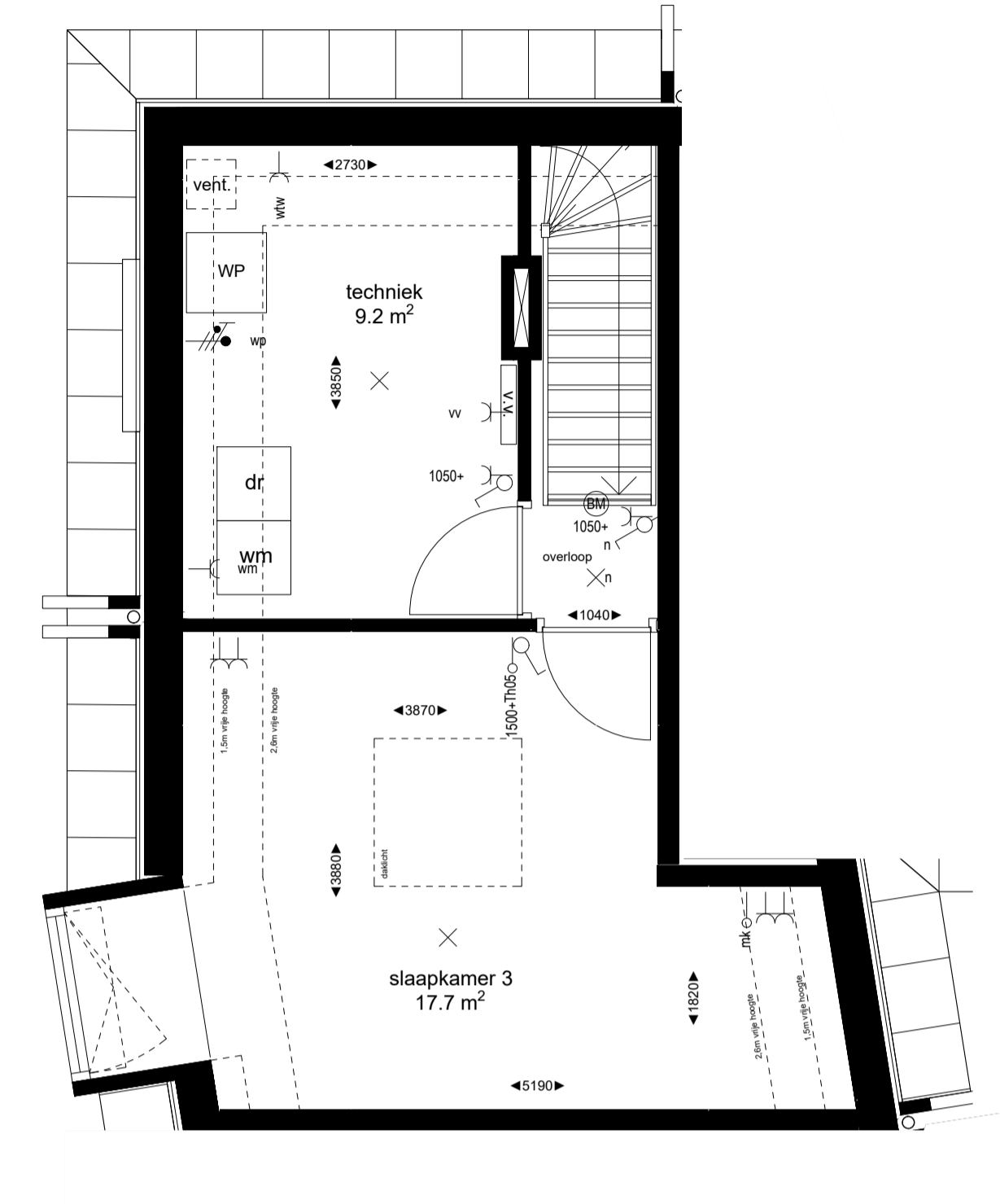
2e verdieping
