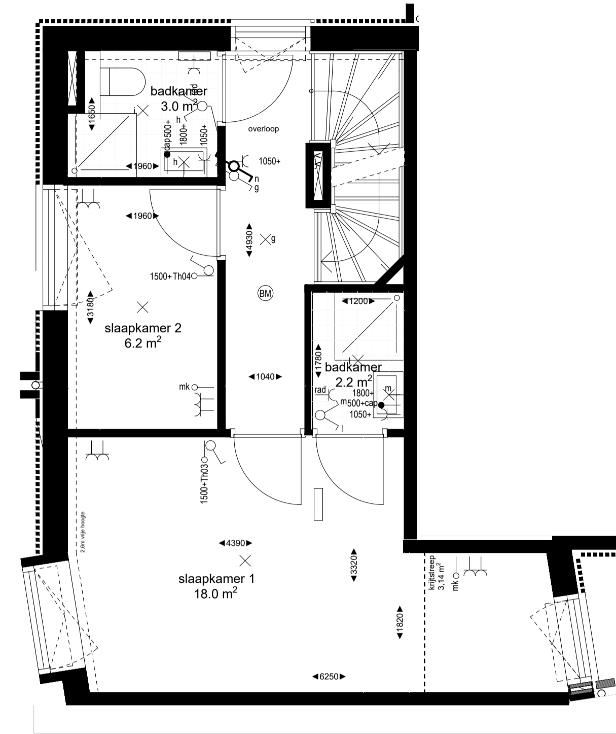
1e verdieping
