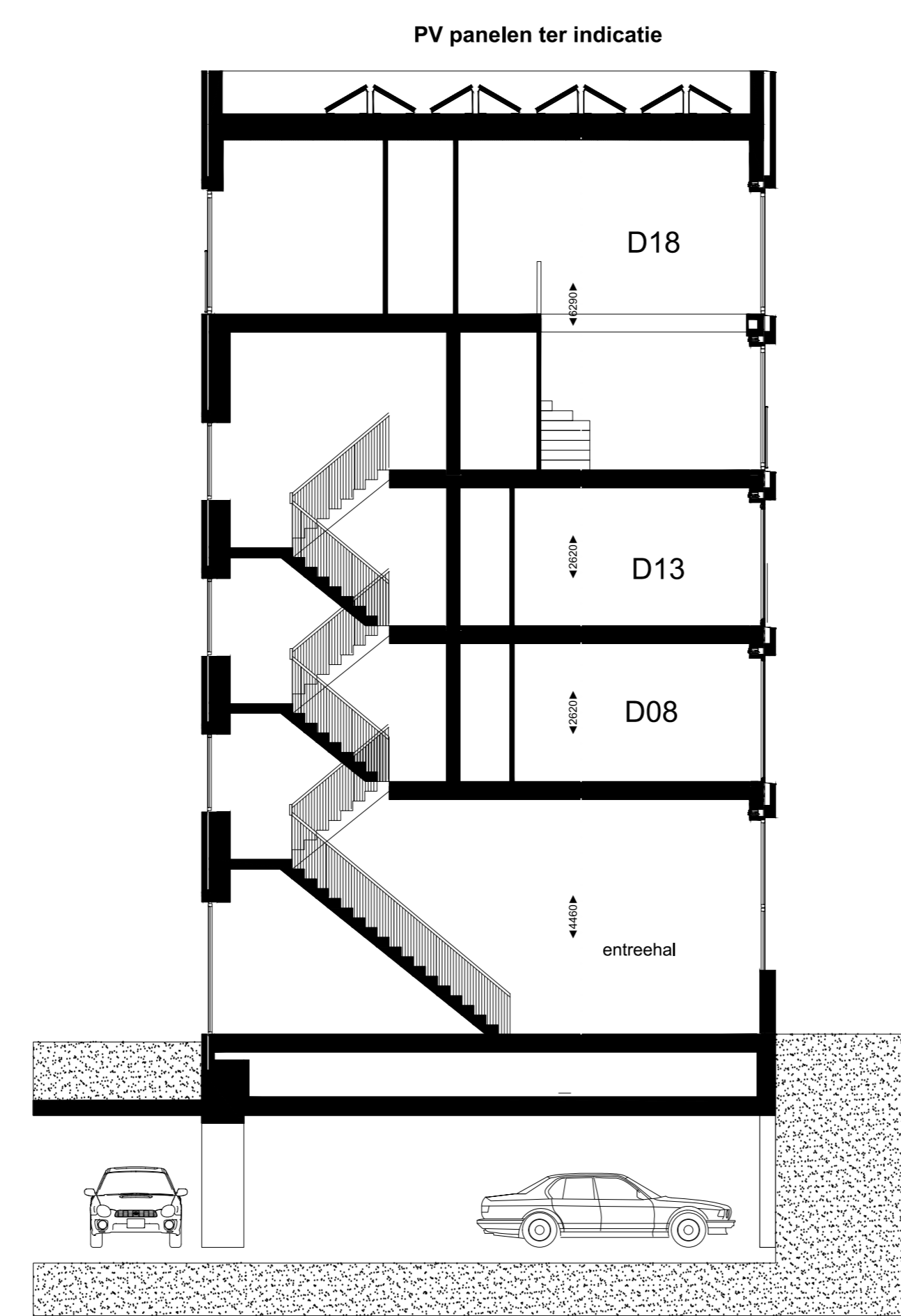
Doorsnede Blok D - de Drie Pakhuizen
