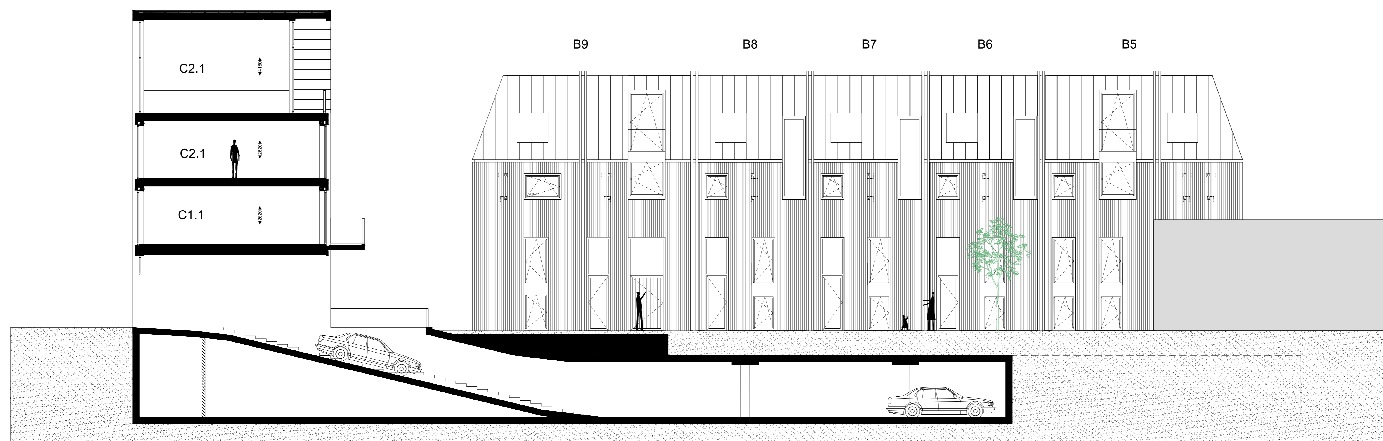
BLOK C - doorsnede het Scheepje
