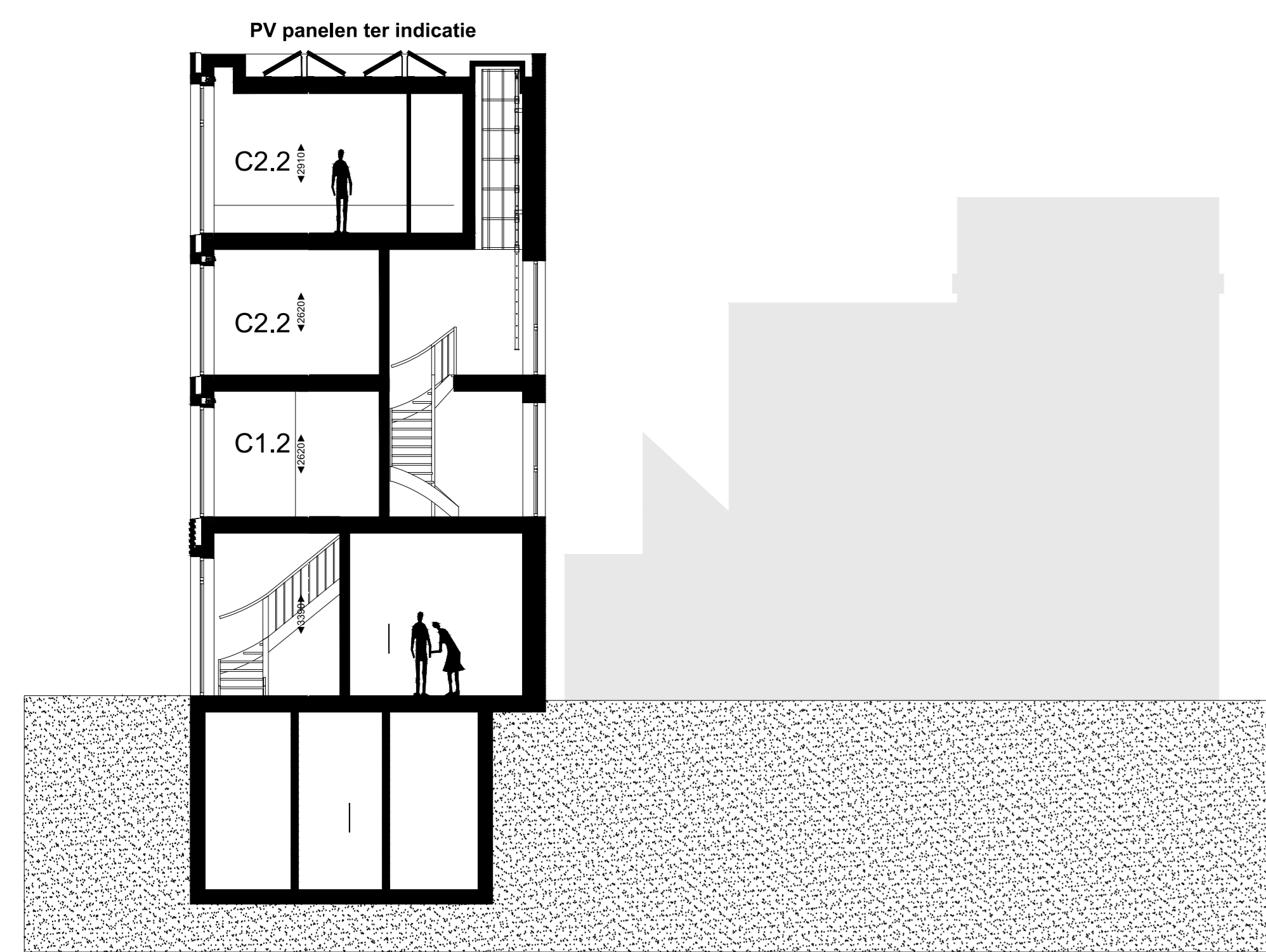
Doorsnede Blok C - het Scheepje
